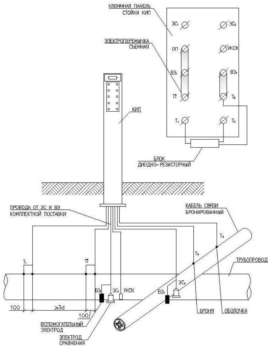
Рисунок Г.4 – Схема подключения КИП на участке пересечения трубопровода с кабелем связи
