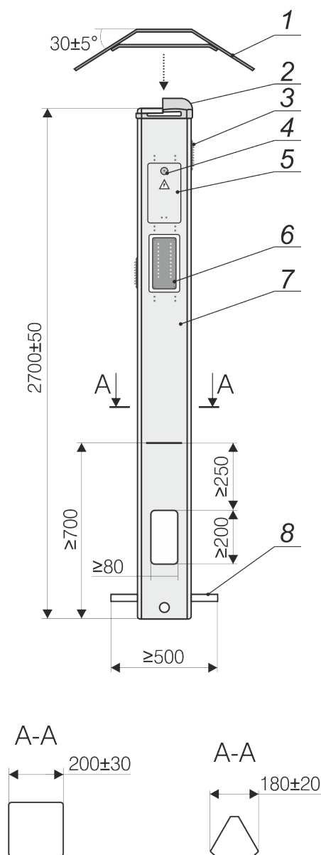
Рисунок А.2 – КИП с люками для открытой установки в грунт над подземным сооружением
