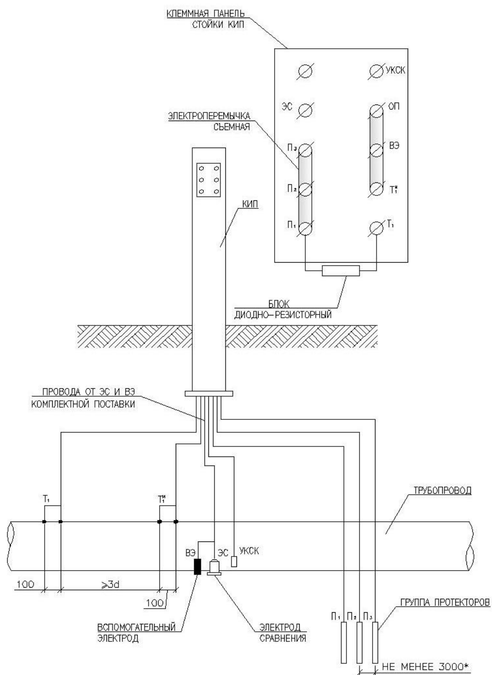
Рисунок Г.2 – Схема подключения КИП на установке протекторной защиты
