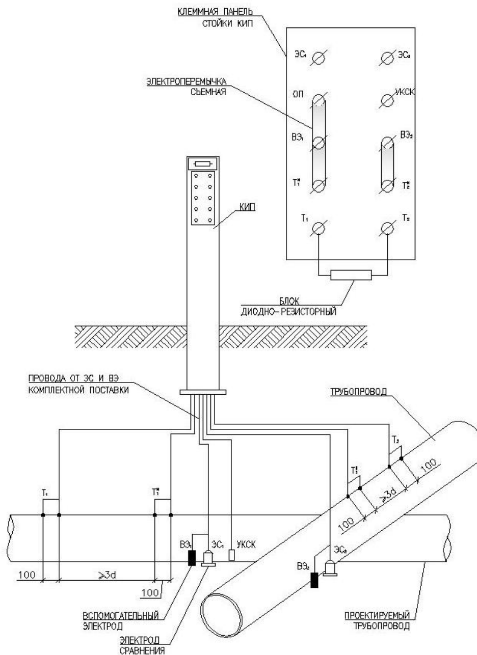
Рисунок Г.3– Схема подключения КИП на участке пересечения двух трубопроводов
