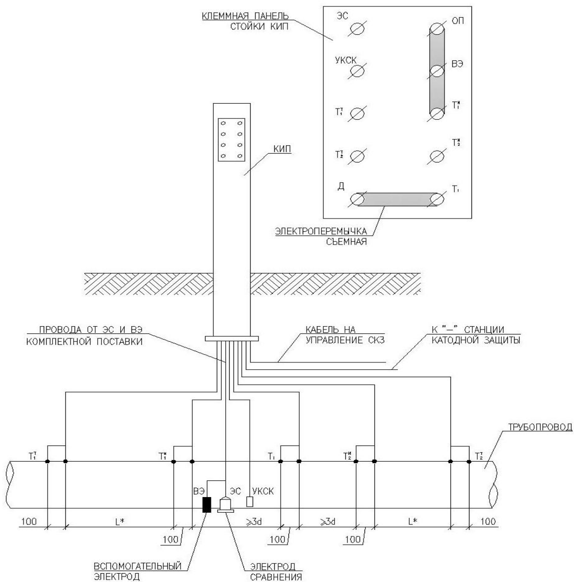
Рисунок Г.1– Схема подключения КИП в точке дренажа
