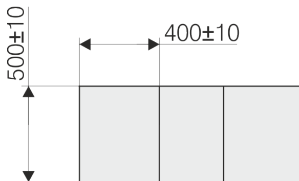
Рисунок А.4 – Километровый знак
