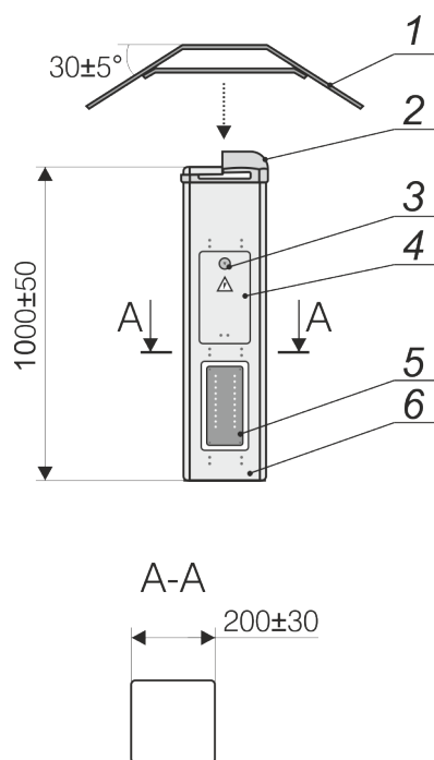
Рисунок А.1 – КИП с люками для открытой установки на надземную часть сооружения
