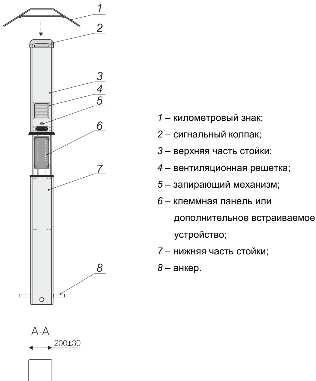
Рисунок А.4 – КИП с люками для открытой установки на надземную часть сооружения
