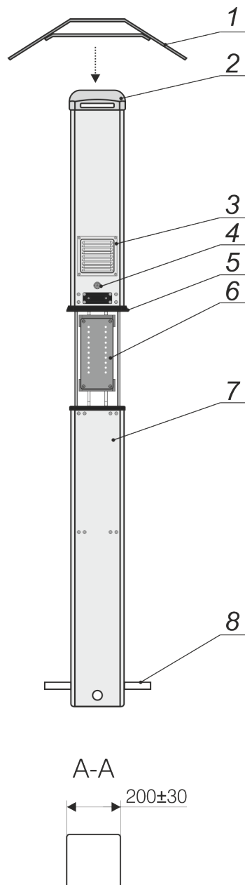
Рисунок А.3 – КИП с подъёмно-раздвижным механизмом для открытой установки в грунт над подземным сооружением
